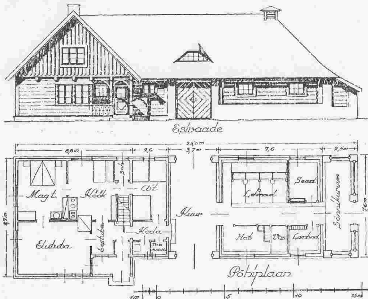
Joon. 24. Elumaja-ait-laut koosehitus: eestvaade ja põhiplaan.
